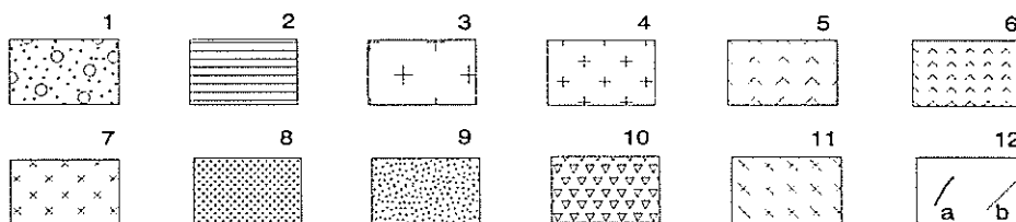
Fig. 7 - Geologia simplificada da área de glaciação da Serra da Estrela. 1 - Depósitos glaciários e fluvioglaciários; 2 - metassedimentos do Complexo Xistograuváquico; 3 - granito de duas micas, porfiróide, de grão grosseiro; 4 - granito de duas micas, porfiróide, de grão médio; 5 - granito moscovítico de grão médio a grosseiro; 6 - granito moscovítico de grão fino; 7 - granito de duas micas de grão médio; 8 - granito orbicular de duas micas, de grão médio; 9 - granito de duas micas, de grão fino; 10 - granito biotítico, de grão fino; 11 - granito biotítico, de grão médio; 12 - a) rochas filoneanas; b) falhas.
