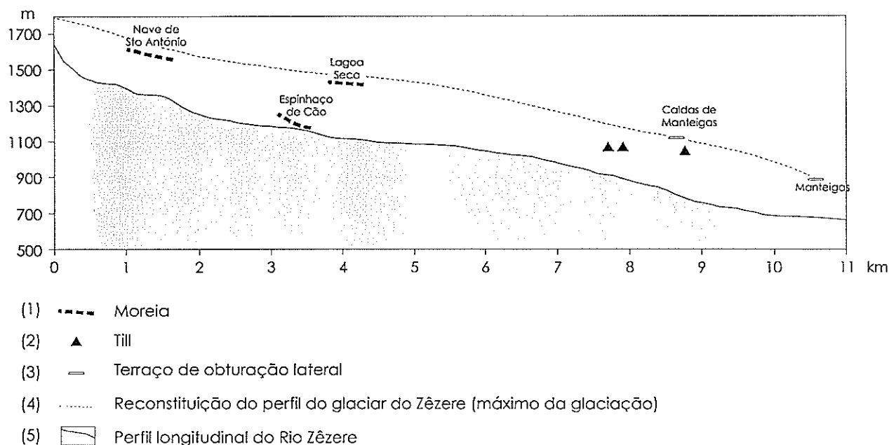
Figura 3 - Depósitos glaciários e reconstituição da língua glaciária do Zêzere.
