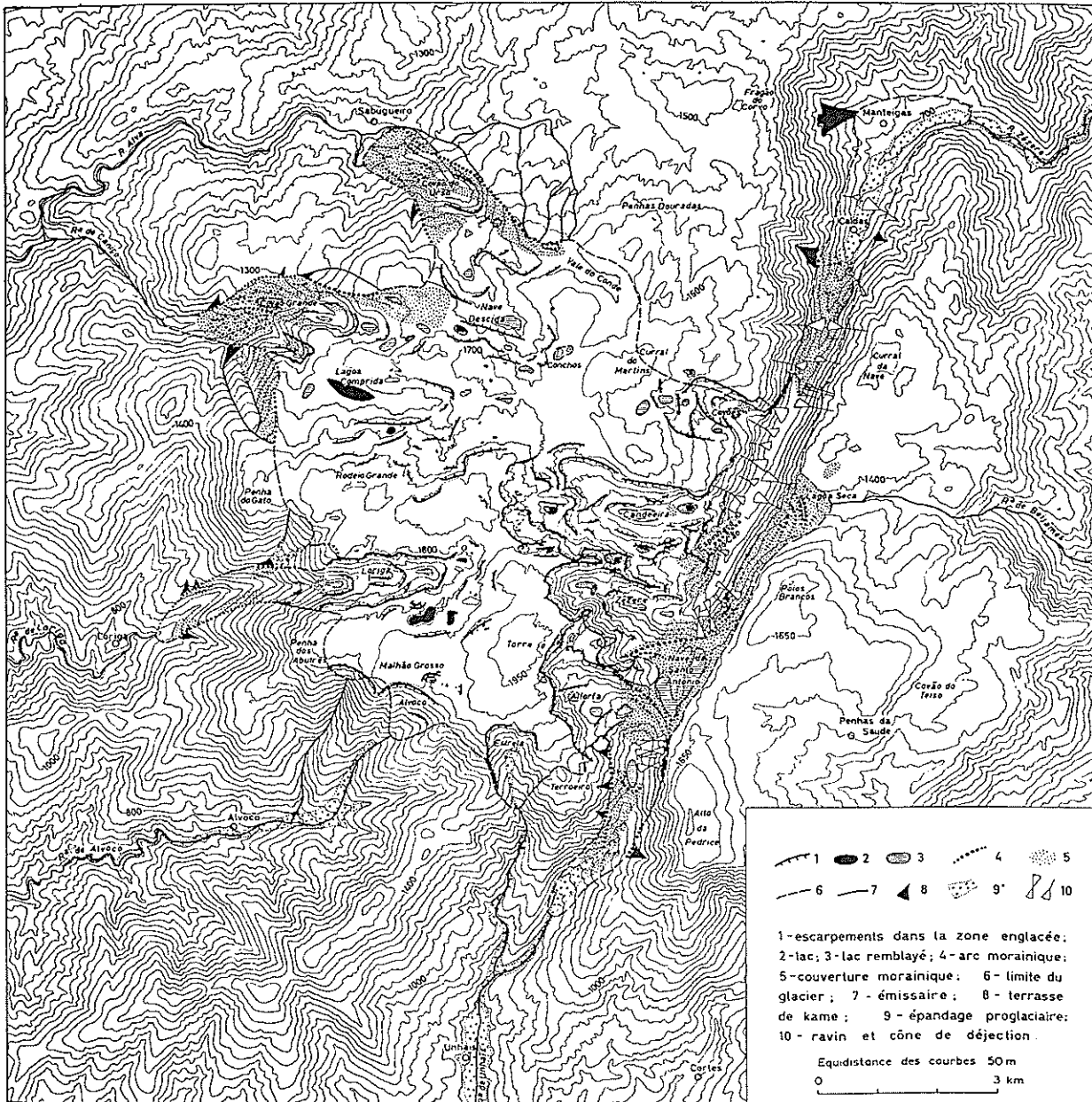
Figura 1 - Glaciação da Serra da Estrela (DAVEAU, 1971). 1 - Escarpas na área da glaciação; 2 - lago; 3 - lago colmatado; 4 - arco morénico; 5 - cobertura morénica; 6 - limite do glaciár; 7 - rio proglaciário; 8 - terraço de obturação lateral; 9 - depósito proglaciário; 10 - barranco e cone de dejeção.
